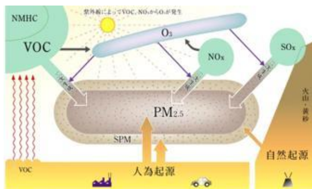
PM2.5の生成メカニズム
