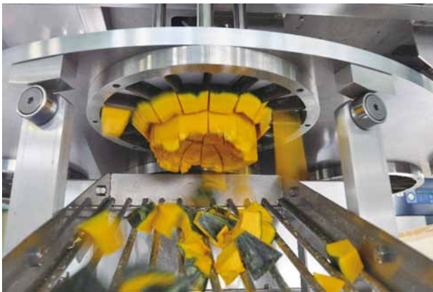
カボチャ乱切り機
