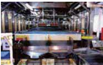
【自動バレルめっき装置】
