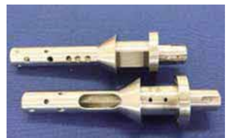
【風洞実験用】
