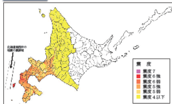
震度分布
