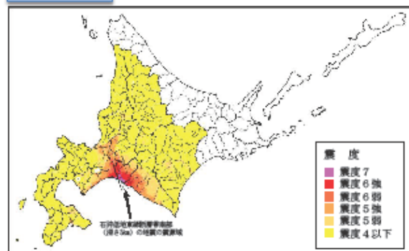
震度分布
