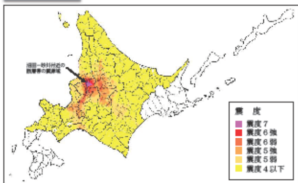
震度分布
