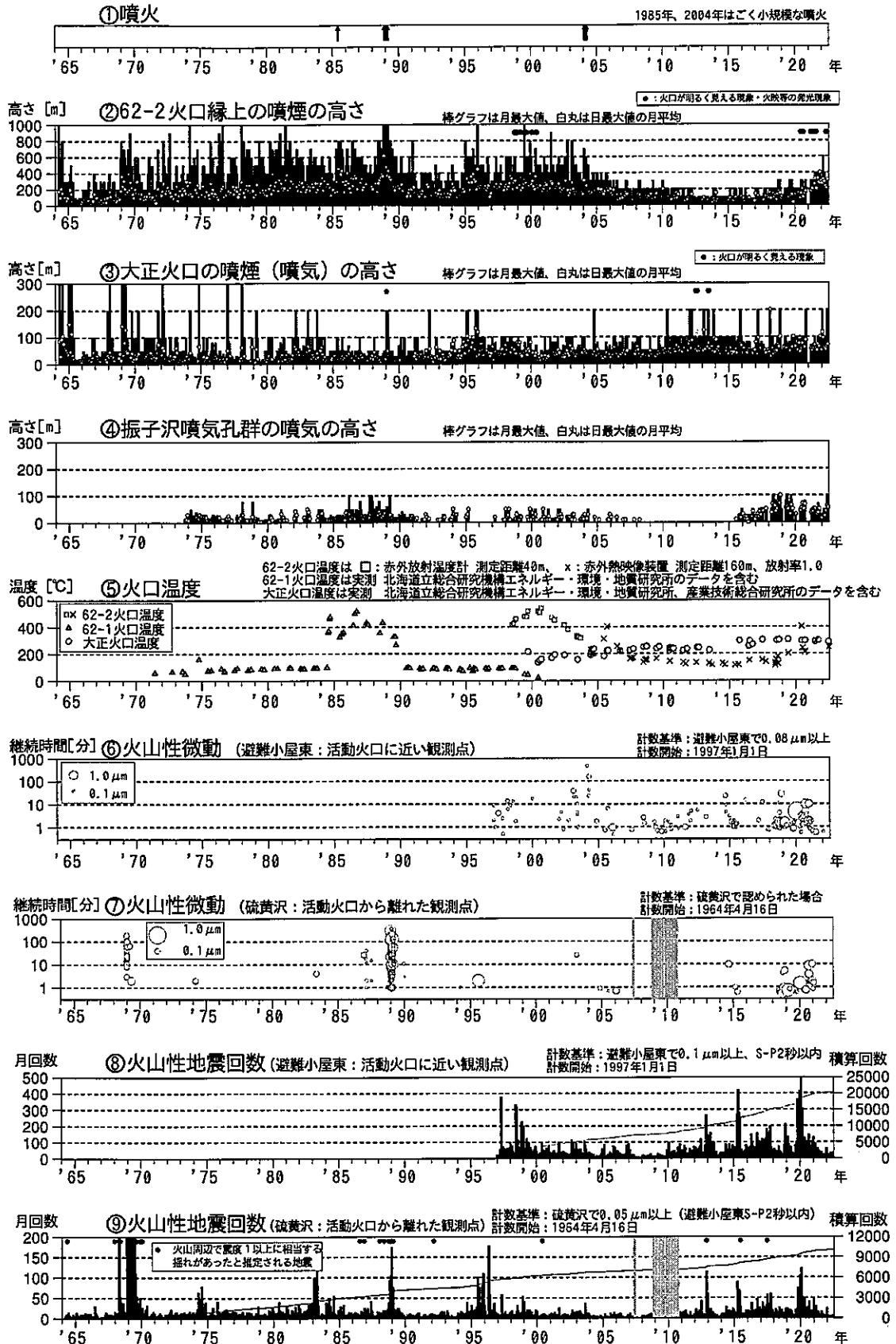
図1 十勝岳 火山活動経過図(1964年1月~2022年7月16日) ⑦⑨: グラフの灰色部分は機器障害による欠測期間を示します。
