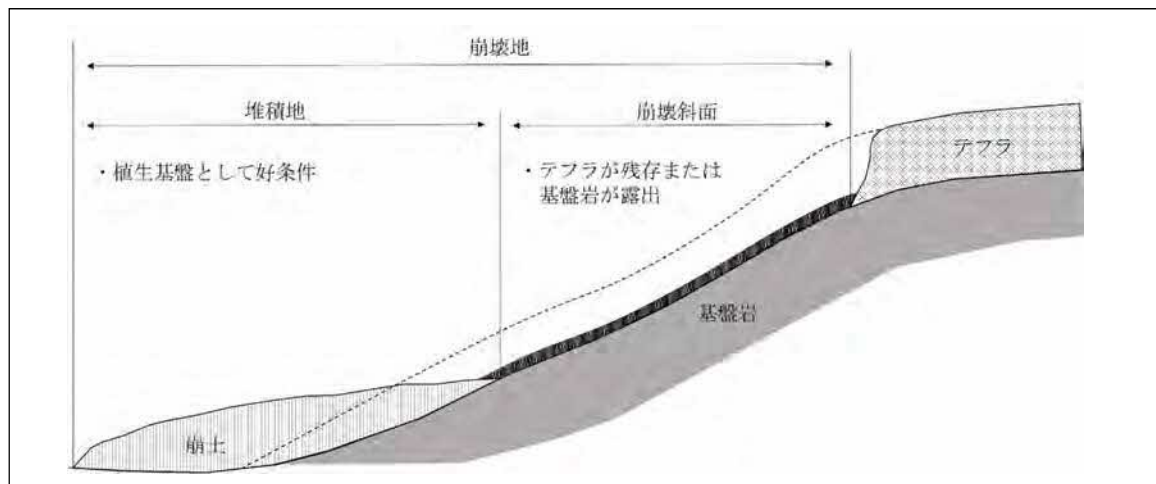
図2. テフラの崩壊模式図
