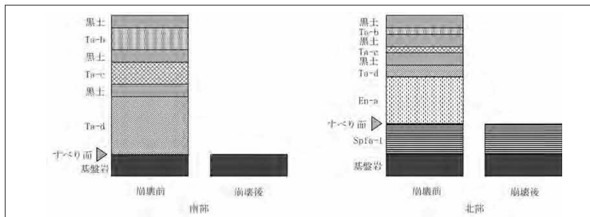
図 4. 地区ごとの崩壊前後の斜面上テフラ模式図 (一例)
