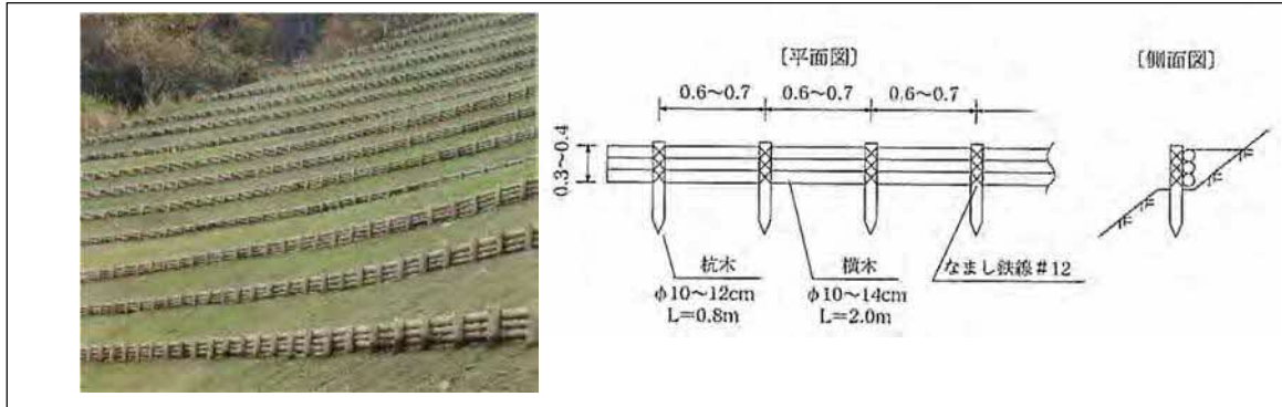
図8. 筋工施工地と施工標準図
