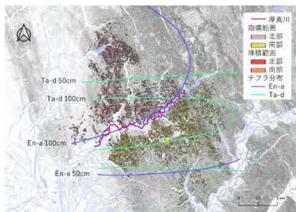
図 3. テフラの等厚分布と崩壊地(林野庁・国土防災技術株式会社 (2020) を基に作成)
