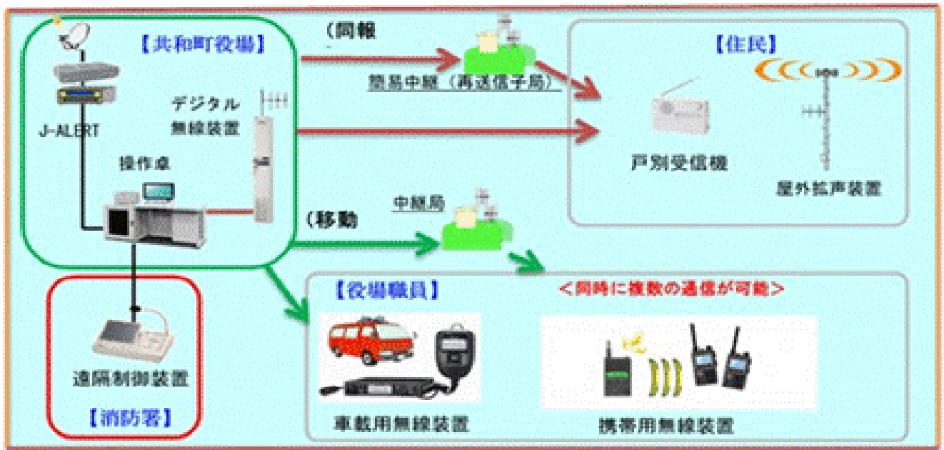
防災行政無線システム図
