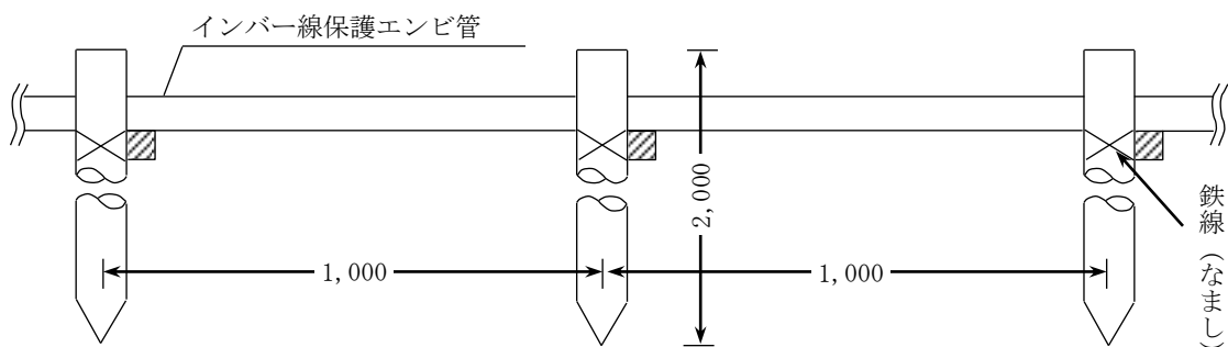
側面図
