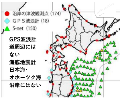
海底地震計・GPS波浪計の設置状況
