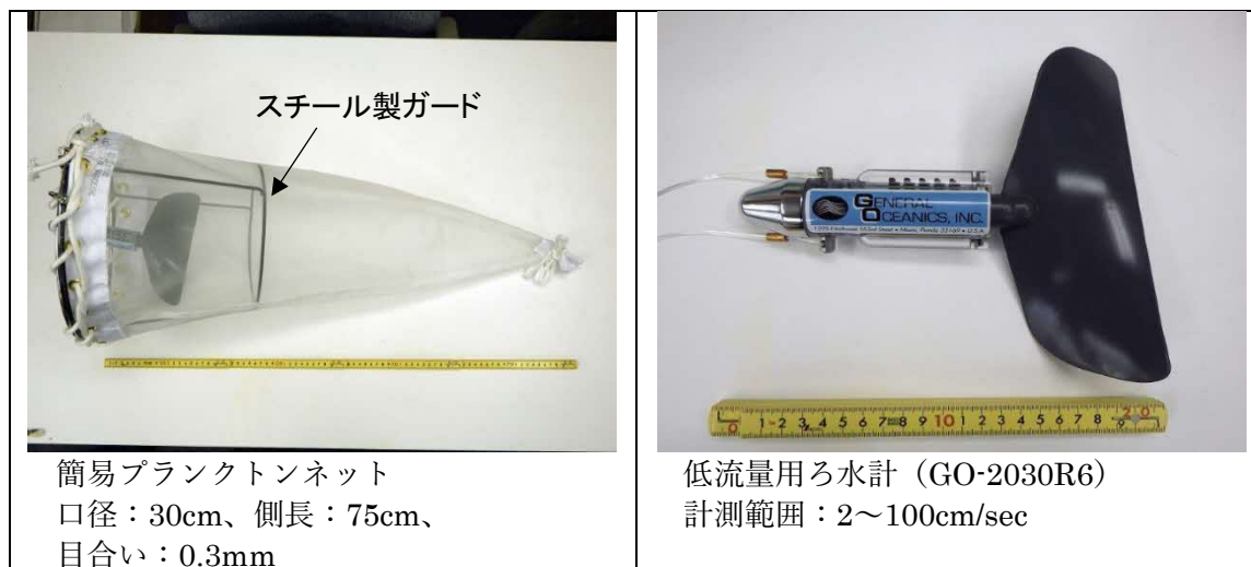
採取器具 (図 3)
