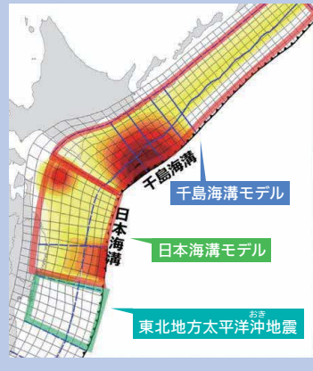
最大クラスの地震・津波を発生させる断層モデル
